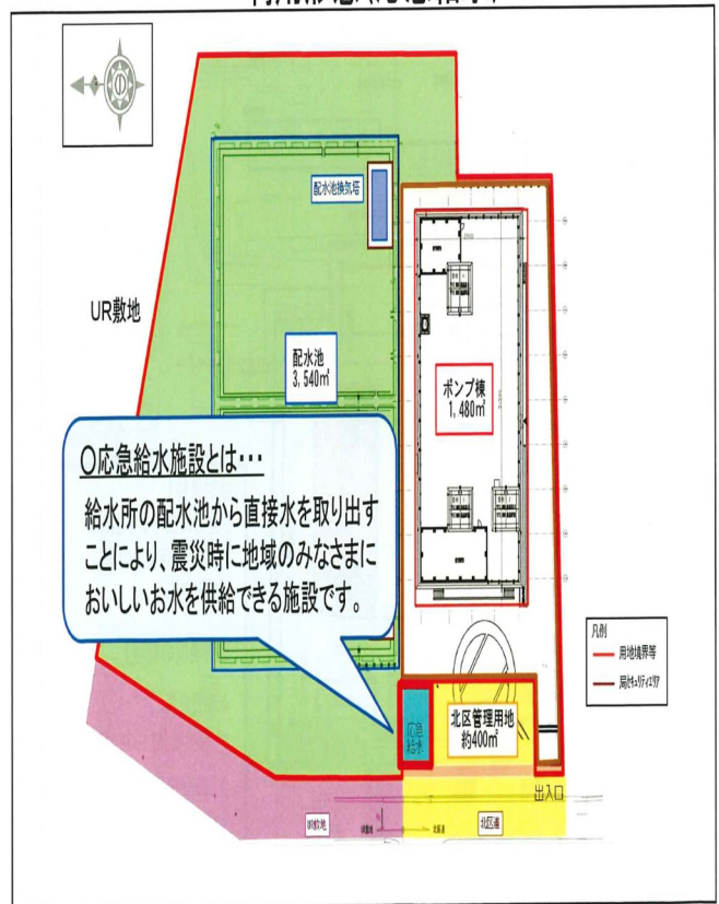
対象敷地 地名地番:王子5丁目1番46 住居表示:王子5丁目2番
